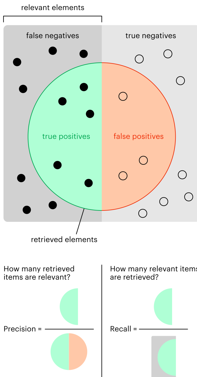
Рис. 8. Визуализация концепции precision
