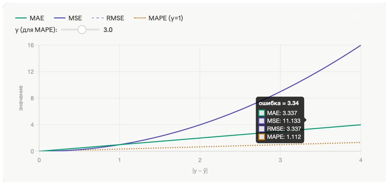
Рис. 4. Значение штрафа метрики в зависимости от размера ошибки. Сгенерировано через Claude
