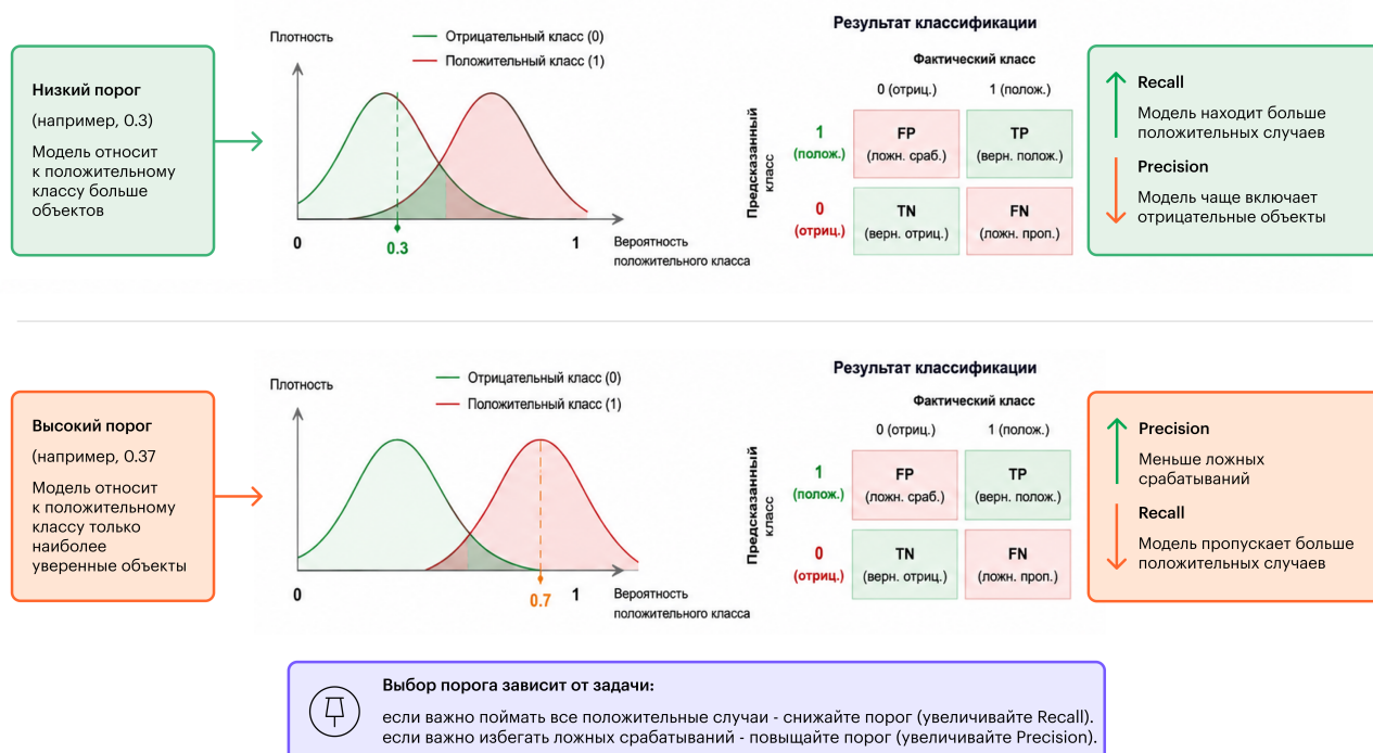
Рис. 10. Изменение порога классификации и его влияние на precision и recall
