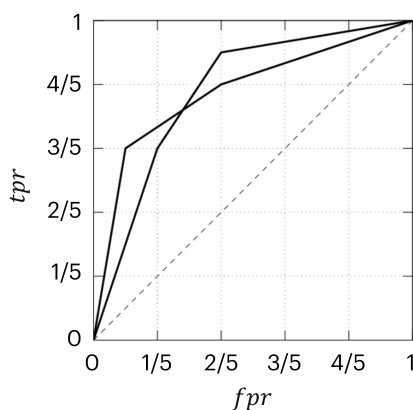
Рис. 21. Разные ROC-кривые, но с одинаковым AUC
