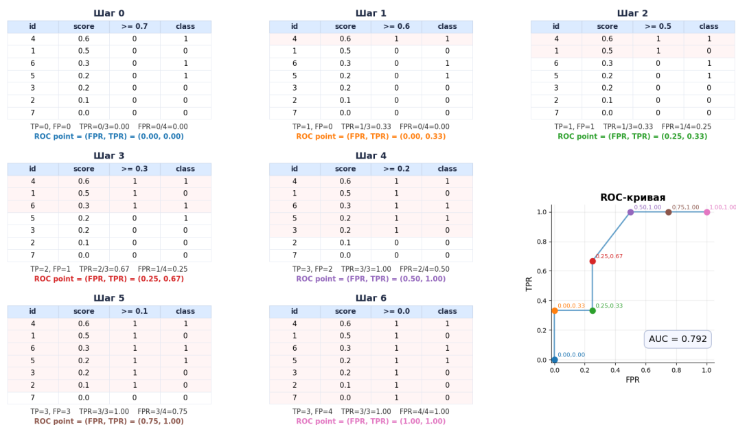
Рис. 20. Пошаговые расчеты построения ROC-кривой
