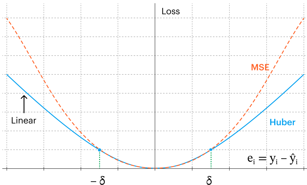
Рис. 2. Визуализация графика Huber loss
