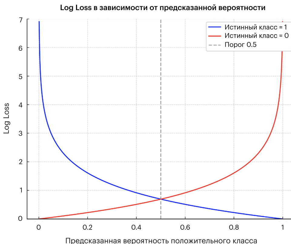
Рис. 6. Log loss в зависимости от предсказанной вероятности
