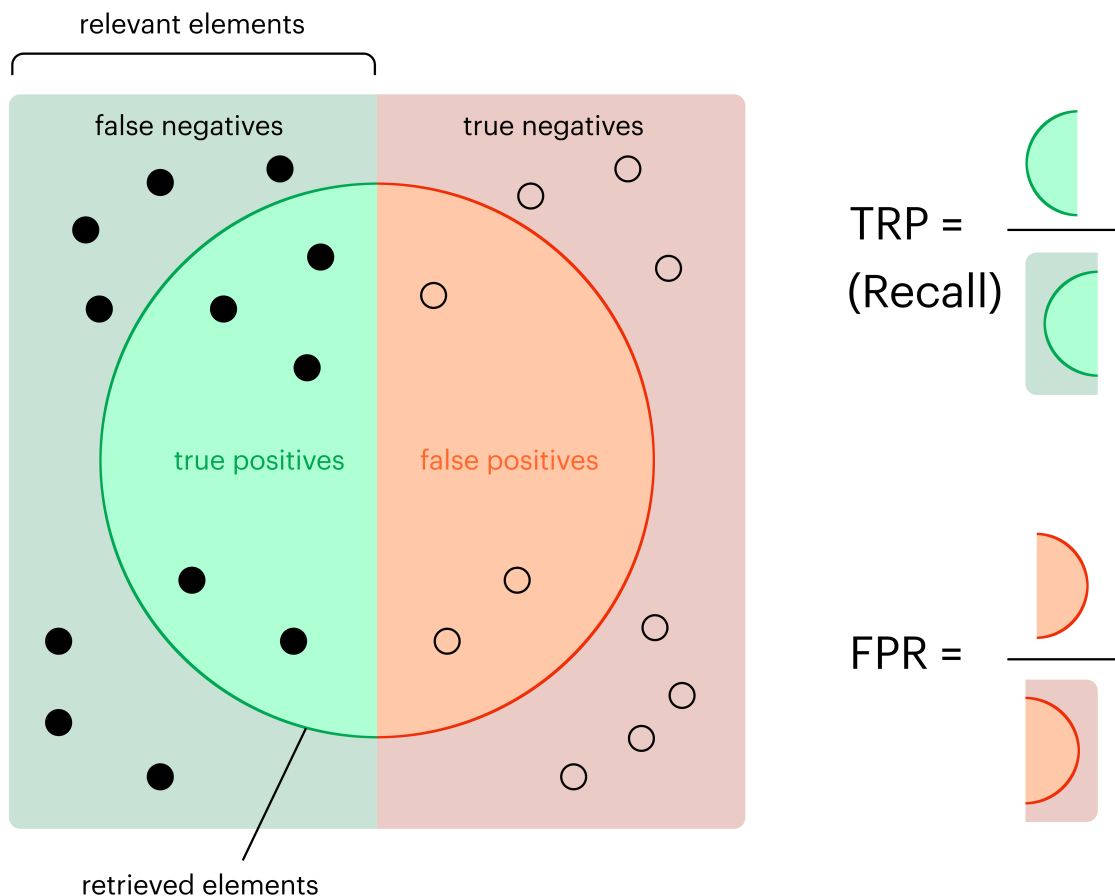
Рис. 14. Метрики true positive rate и false positive rate
