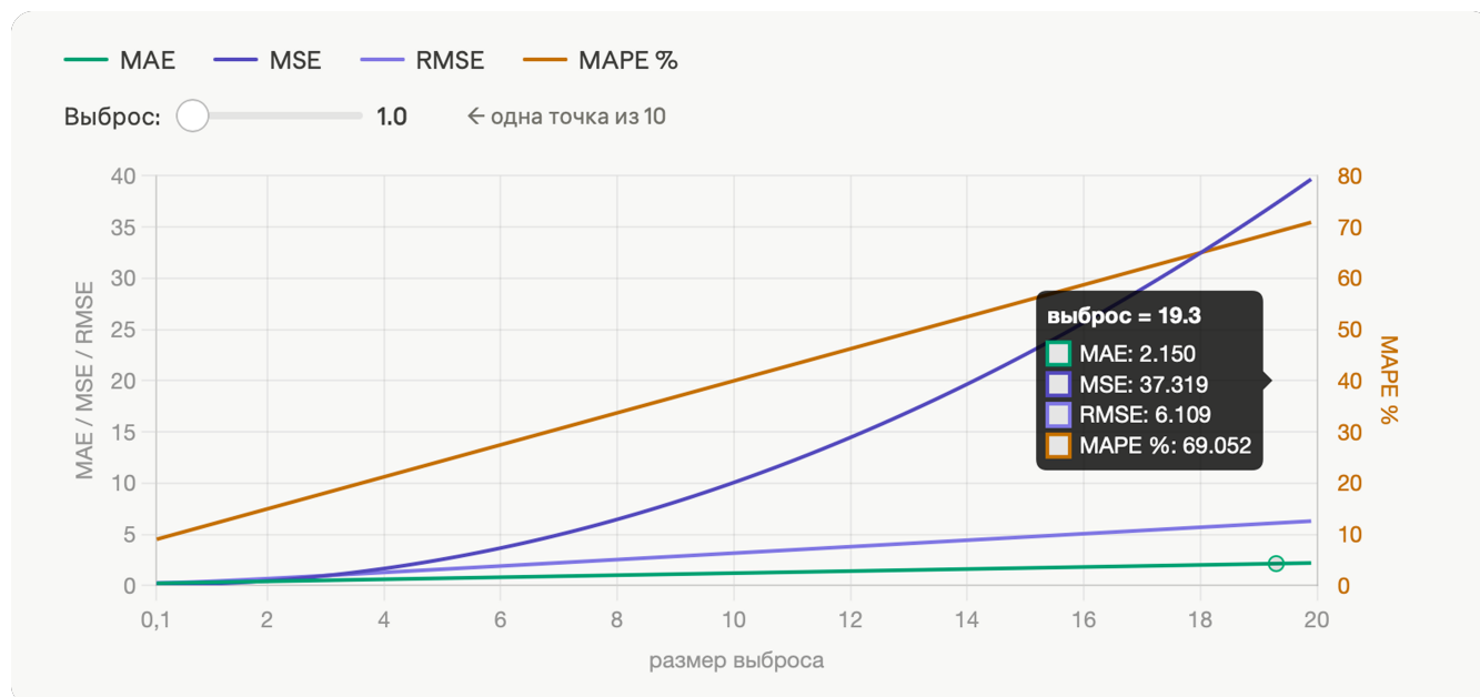
Рис. 5. Влияние выброса на поведение метрики. Сгенерировано через Claude
