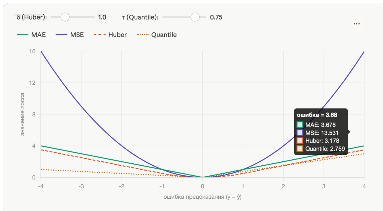
Рис. 3. Визуализация штрафов за ошибки разного размера для loss-функций — MAE, MSE, Huber loss, quantile loss.
