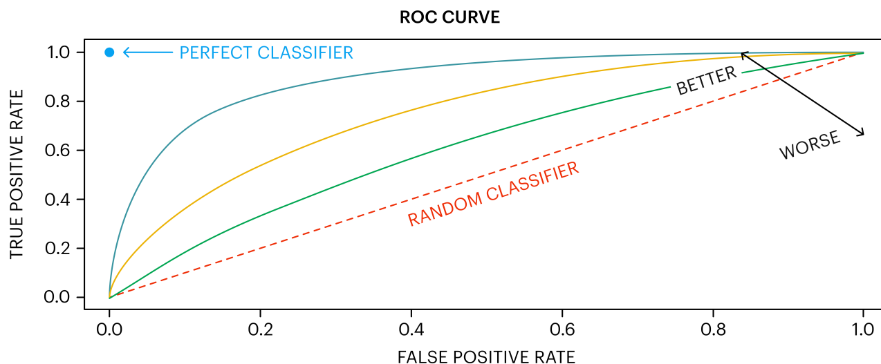
Рис. 15. Визуализация различных ROC-кривых
